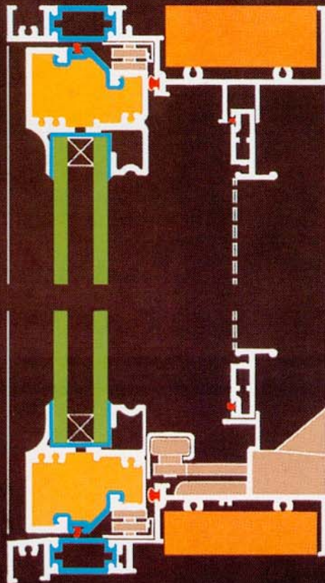
coupe verticale
